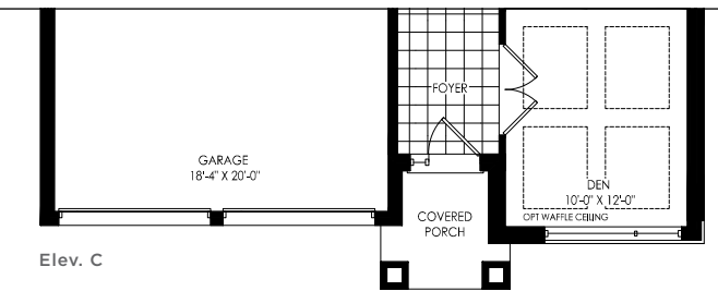
Elev. C
